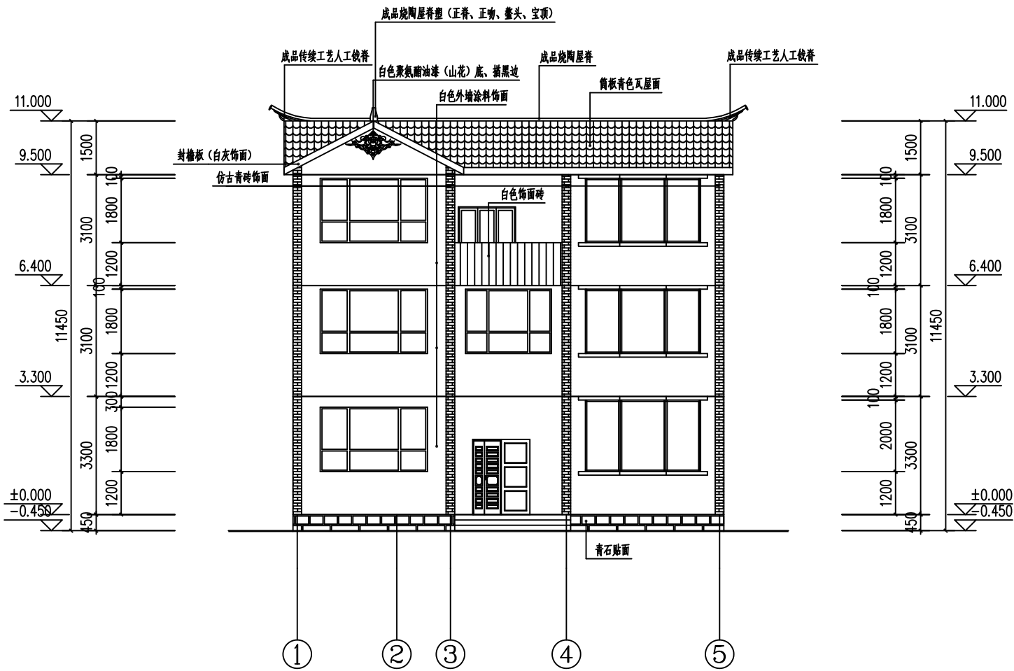
①-⑤轴立面图 1:100
